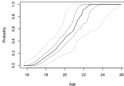
Population posterior
